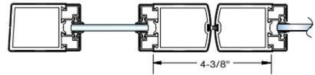
Offset Hung Door
