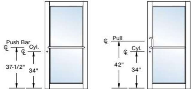
Center Hung Door
