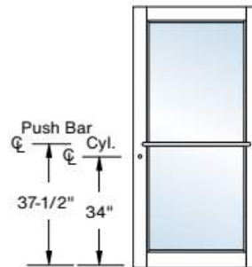
Center Hung Door
