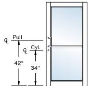
Offset Hung Door
