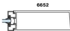
Offset Hung Door
