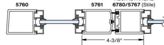
Offset Hung Door
